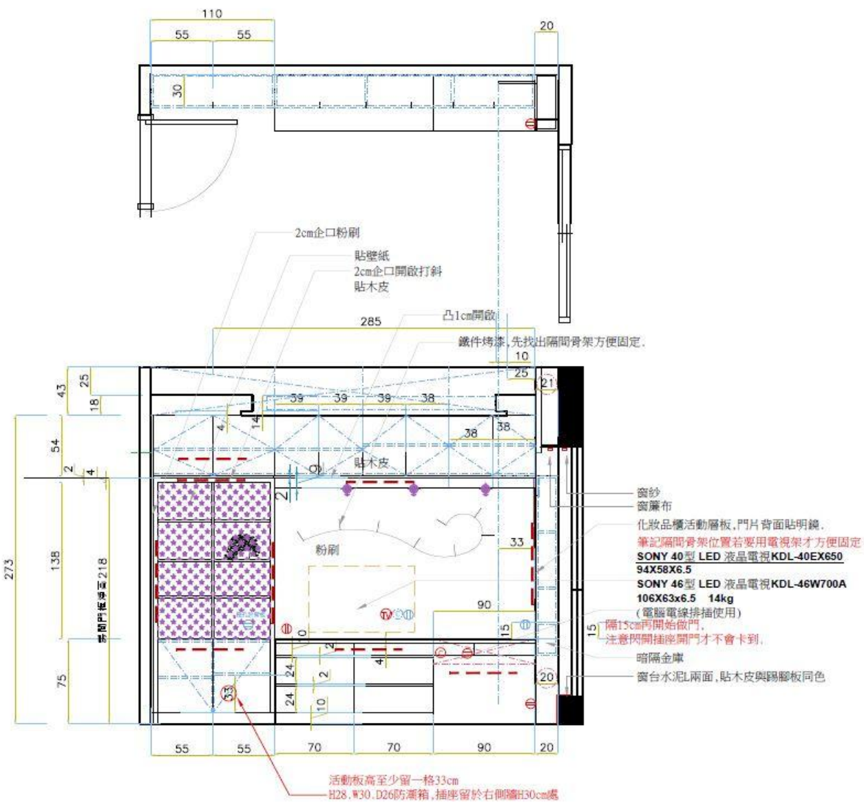
10 主臥電視牆立面圖
