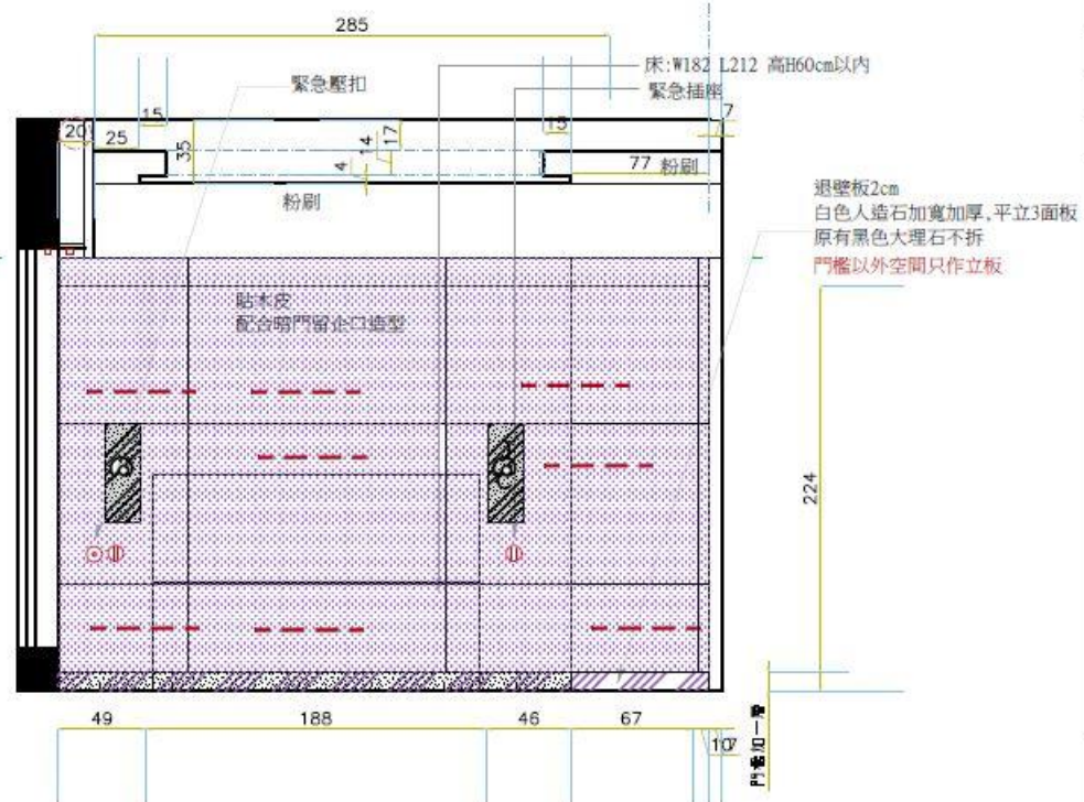
11 主臥主牆浴暗門立面圖
