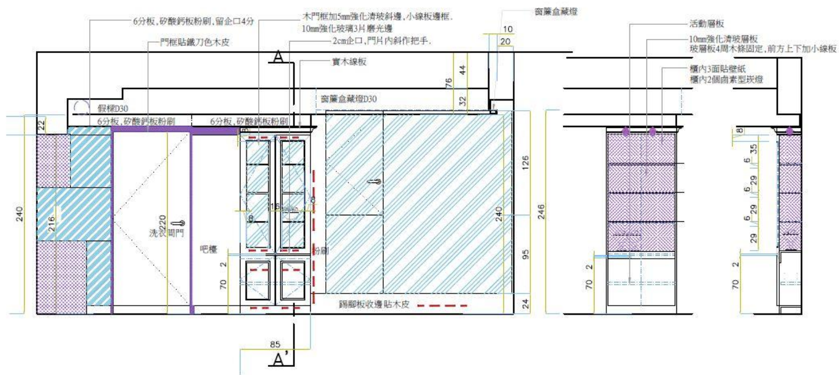
03 餐廳窗邊高櫃立面圖
