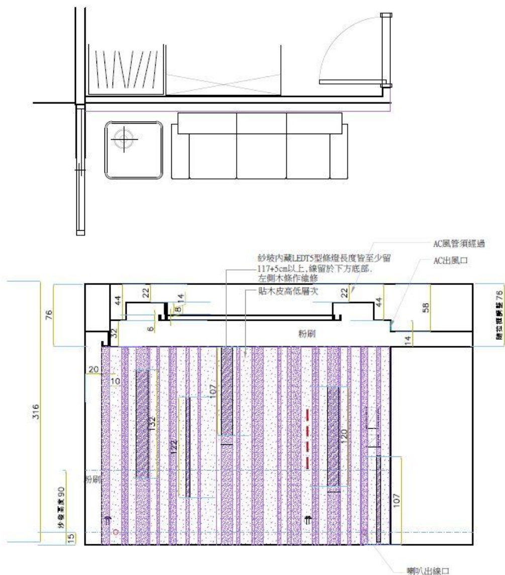
05 客廳沙發主牆立面圖
