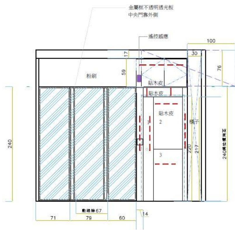
12 主臥更衣室拉門立面圖
