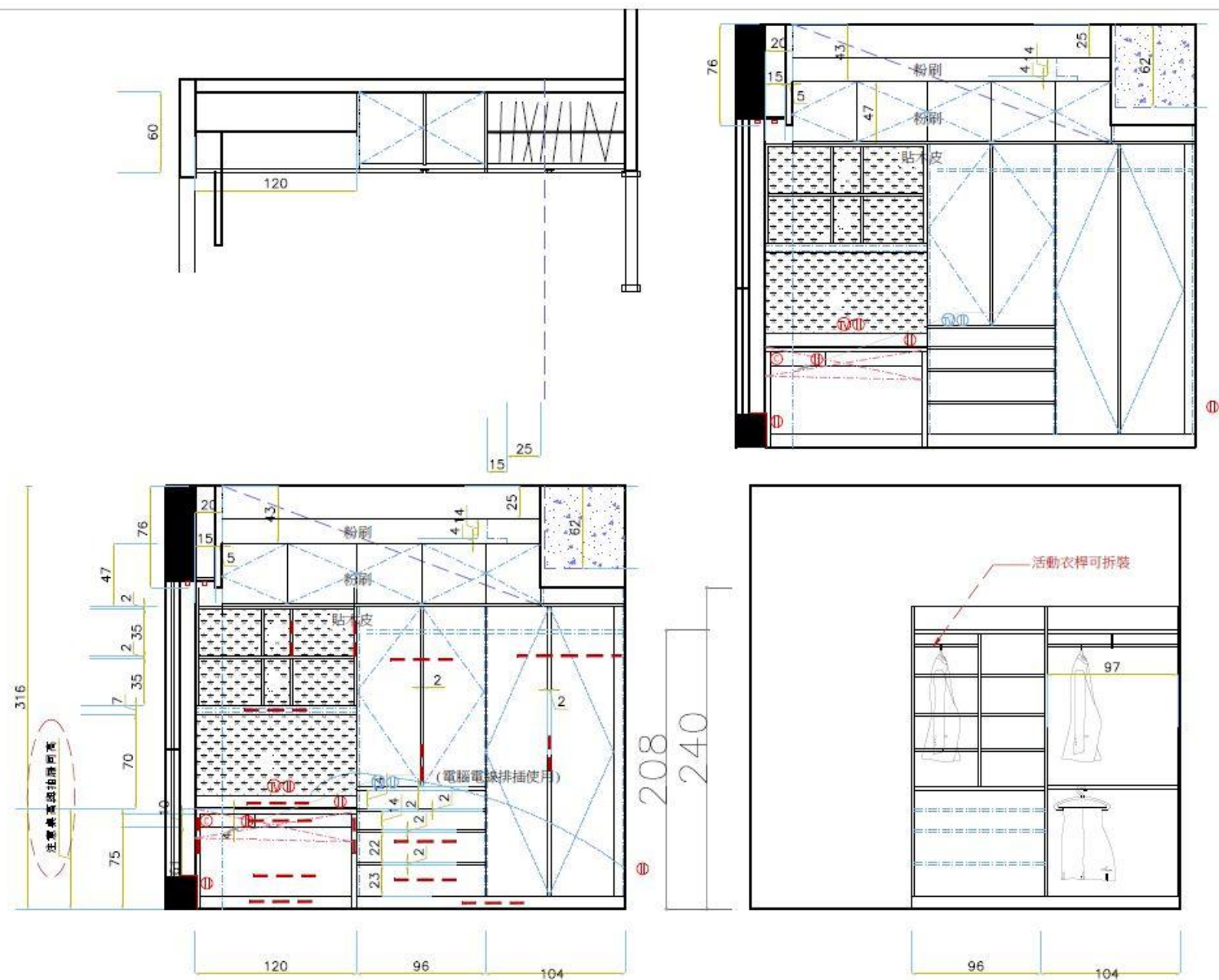
16 臥A衣櫃立面圖
